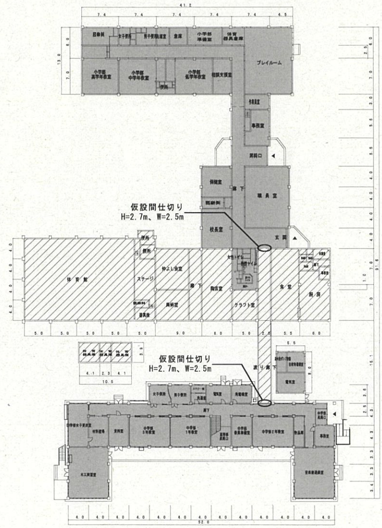
平面図 S=1 : 500
